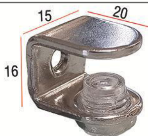
descrizione: MORSETTO TONDO codice: 8608507 misura: L.15 x P.20 x H.16 mm - vetri max 10 mm finitura: nichelato
