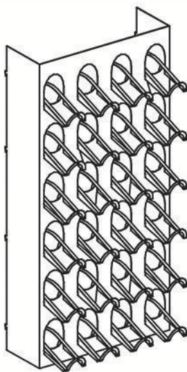
P/BOTTIGLIE PER MONTANTE MODULO INFERIORE
