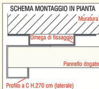
Finitura con zoccolo alto (h.15 cm) inf. e sup. e profilo a C ai lati di ogni pannello - H=270 cm
