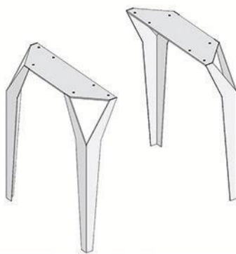
descrizione: COPPIA GAMBE INDUSTRIAL codice: BK-CPGB.IND72 misura: L.14 x P.50 x H.72 cm finitura: bianco RAL9010 / nero RAL9004
