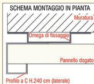
Finitura con profilo a C ai lati di ogni pannello H=240 cm
