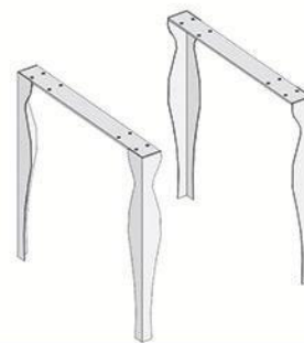
descrizione: COPPIA GAMBE SHABBY codice: BK-CPGB.SH50 misura: L.8 x P.50 x H.50 cm finitura: bianco RAL9010 / nero RAL9004
