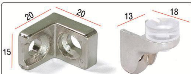
descrizione: REGGIPIANO R/VETRO CON GOMMINO codice: 8072507 8045007 misura: L.1,5 x P.2 x H.2 cm L.1,3 x P.1,8 x H.2 cm finitura: nichelato nichelato
