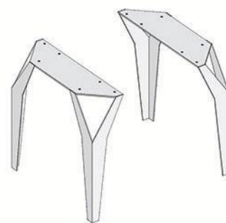
descrizione: COPPIA GAMBE INDUSTRIAL codice: BK-CPGB.IND50 misura: L.14 x P.50 x H.50 cm finitura: bianco RAL9010 / nero RAL9004
