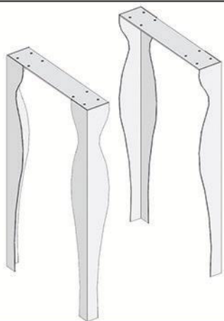
descrizione: COPPIA GAMBE SHABBY codice: BK-CPGB.SH90 misura: L.10 x P.50 x H.90 cm finitura: bianco RAL9010 / nero RAL9004
